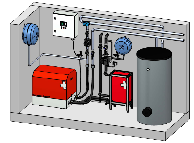
ISOMETRIE
